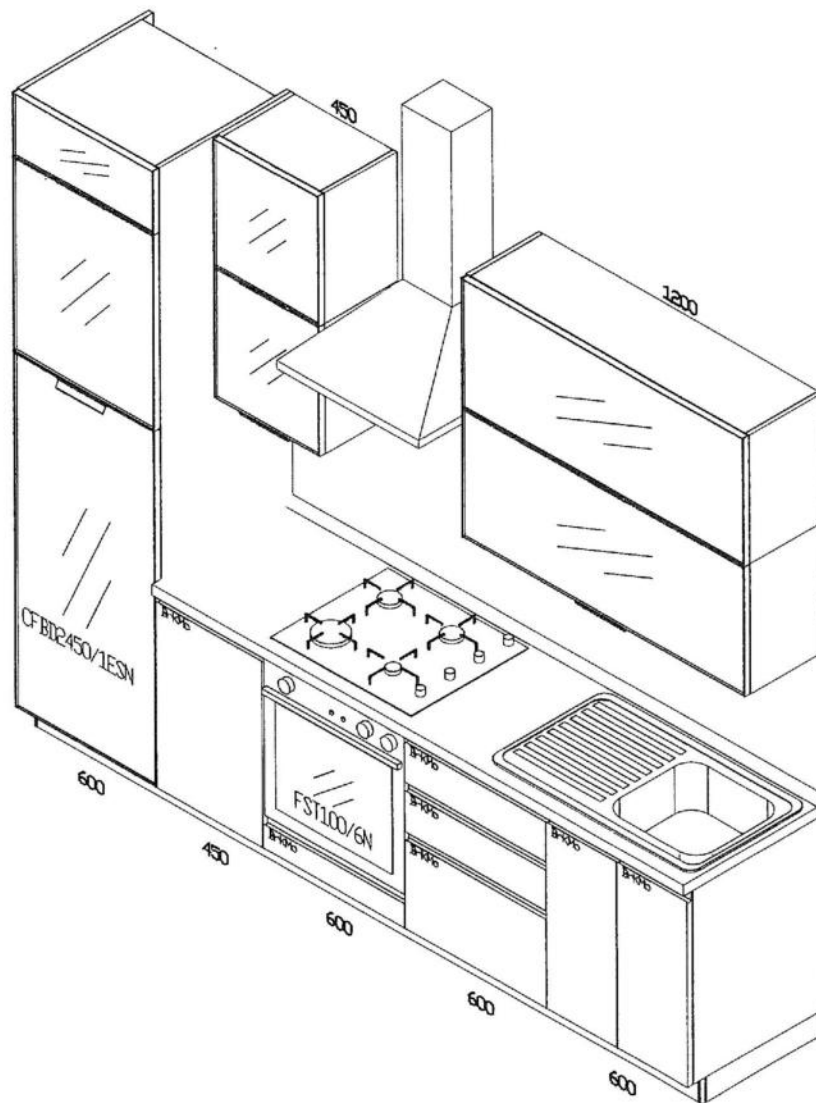
Assonometria
